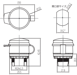
RJ45 プラグポート
