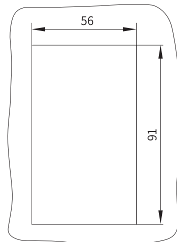
カットアウト寸法 (このページの製品に適用)
