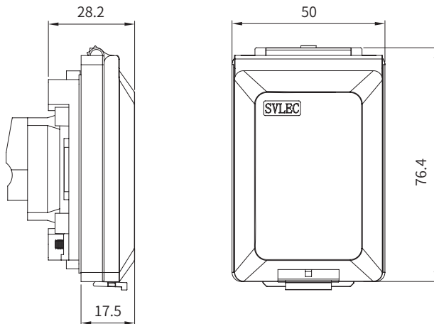
全体寸法
