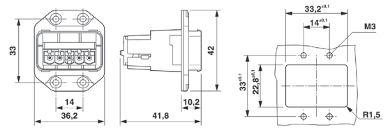
プッシュプル式電源ハウジング
