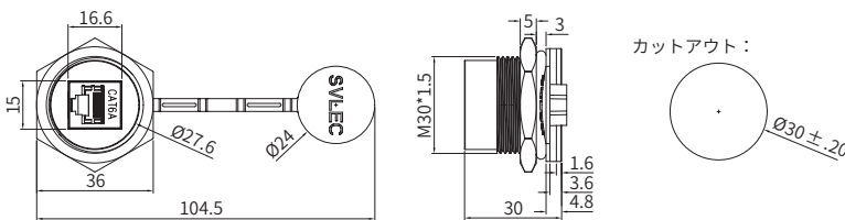
RJ45 防水コネクタ
