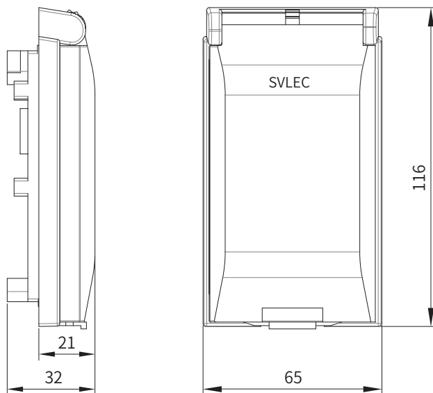
全体寸法
