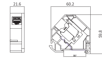
プッシュプル式 RJ45 コネクタ
