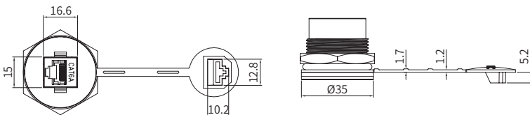
RJ45 ポートアダプター CAT6A
