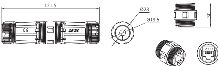
RJ45 防水コネクタ
