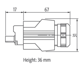
プッシュプル式電源コネクタ
