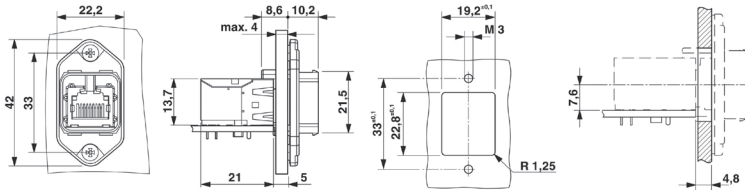
RJ45 コネクタハウジング
