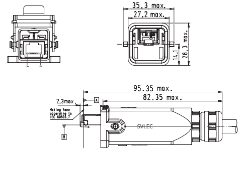
RJ45 オス
