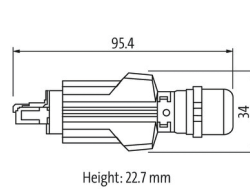
プッシュプル式 RJ45 コネクタ
