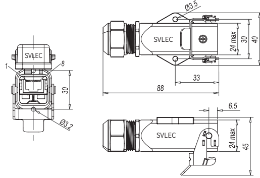
RJ45 フード
