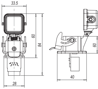
RJ45 ハウジング
