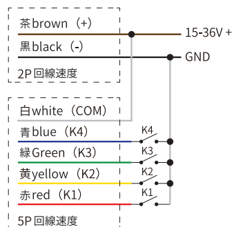
図1 プラスコモン NPN
