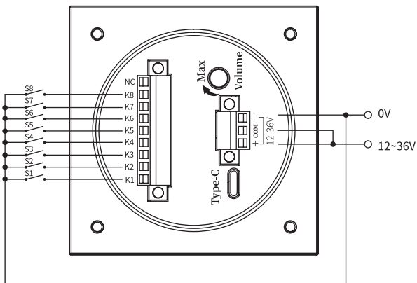
図 1NPN 方式
