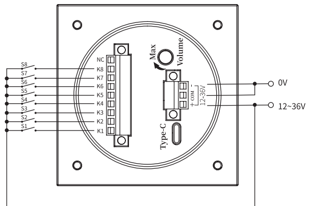
図 2PNP 方式
