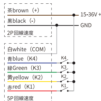
図2 マイナスコモン PNP
